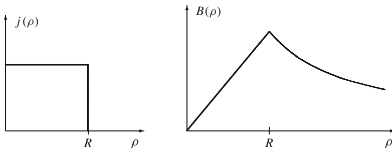
Abbildung 14.1 Stromverteilung \mathbf{j} = j(\rho) \mathbf{e}_z und Feldstärke \mathbf{B} = B(\rho) \mathbf{e}_\varphi eines homogen durchflossenen Drahts.
