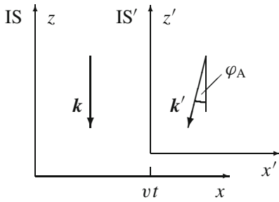
Abbildung 22.4 Eine ebene Welle mit dem Wellenvektor k in IS hat in IS' einen etwas anders gerichteten Wellenvektor k' . Hiermit kann die Aberration erklärt werden: Die Bahnbewegung der Erde um die Sonne führt dazu, dass sich ein bestimmter Stern auf einem kleinen Kreis zu bewegen scheint.
