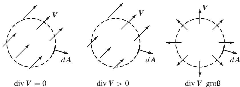
Abbildung 1.2 Zur Berechnung der Divergenz (1.2) wird ein kleines Volumen \Delta \mathcal{V} betrachtet (hier speziell kugelförmig). Wenn das Vektorfeld \mathbf{V} im Bereich des Volumens konstant ist (links), verschwindet die Divergenz. Nimmt \mathbf{V} dagegen in Feldrichtung zu (Mitte), so ist \text{div } \mathbf{V} positiv. Die Divergenz wird maximal, wenn das Vektorfeld durchweg parallel zum Flächenvektor d\mathbf{A} der Oberfläche von \Delta \mathcal{V} ist (rechts). Das Vektorfeld hat hier eine Quelle; allgemein ist \text{div } \mathbf{V} ein Maß für die Quellstärke des Felds.
