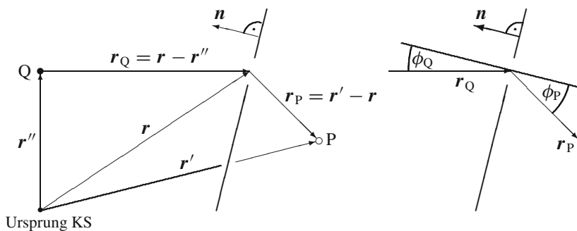
Abbildung 35.2 Ergänzend zu Abbildung 35.1 werden einige Vektoren und Winkel definiert, die in der Rechnung auftreten. Der Vektor \mathbf{r} zeigt zu einem Punkt der Blendenöffnung, \mathbf{r}'' gibt den Ort der Quelle an, \mathbf{n} ist ein Einheitsvektor, der senkrecht auf der Fläche steht. Bei \mathbf{r}' soll das Wellenfeld berechnet werden. Für die im rechten Teil definierten Winkel gilt \mathbf{n} \cdot \mathbf{r}_Q = -r_Q \cos \phi_Q und \mathbf{n} \cdot \mathbf{r}_P = -r_P \cos \phi_P .
