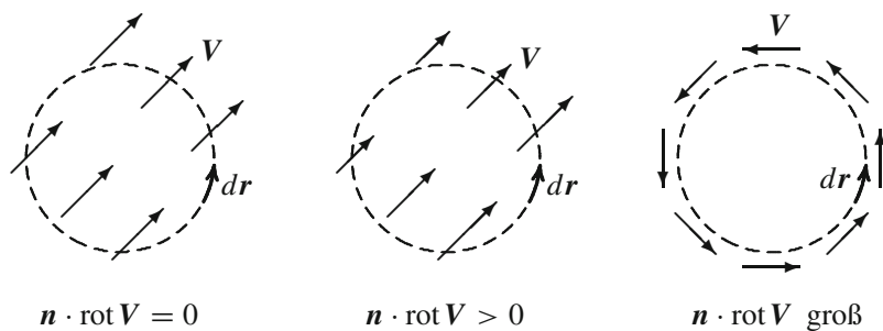
Abbildung 1.3 Zur Berechnung der Rotation (1.3) wird eine kleine Fläche \Delta A (hier speziell kreisförmig) mit dem Normalenvektor \mathbf{n} (senkrecht zur Bildebene) betrachtet. Wenn das Vektorfeld \mathbf{V} im Bereich der Fläche konstant ist (links), verschwindet die Rotation. Nimmt \mathbf{V} dagegen quer zur Feldrichtung zu (Mitte), so ist \mathbf{n} \cdot \text{rot } \mathbf{V} ungleich null. Die Rotation wird maximal, wenn das Vektorfeld durchweg parallel zum Wegelement d\mathbf{r} des Rands von \Delta A ist (rechts). Das Vektorfeld hat hier einen Wirbel; allgemein ist |\text{rot } \mathbf{V}| ein Maß für die Wirbelstärke des Felds.
