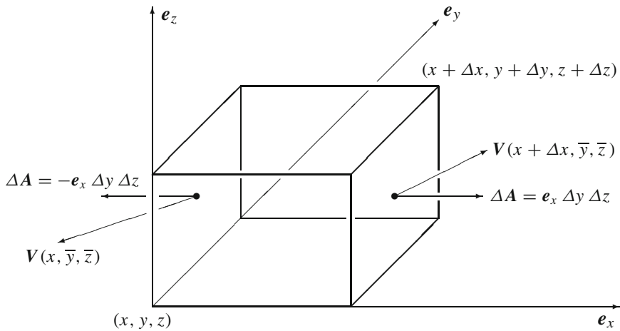
Abbildung 1.4 Zur Berechnung von \text{div } \mathbf{V} in kartesischen Koordinaten wird ein quaderförmiges Volumen \Delta \mathcal{V} = \Delta x \Delta y \Delta z gewählt. Die Beiträge aller sechs Seitenflächen zum Flächenintegral \oint d\mathbf{A} \cdot \mathbf{V} werden aufsummiert und durch \Delta \mathcal{V} geteilt.
